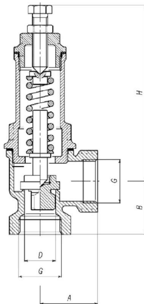
VERSIONE SEDE METALLICA
