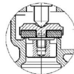
VARIANTE SEDE TEFLON
