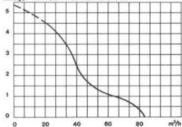
mm H 2 O VENTOLA Ø 96 inclinazione 26°
