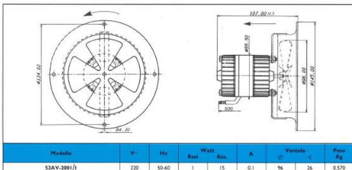
mm H 2 O VENTOLA Ø 96 inclinazione 26°
