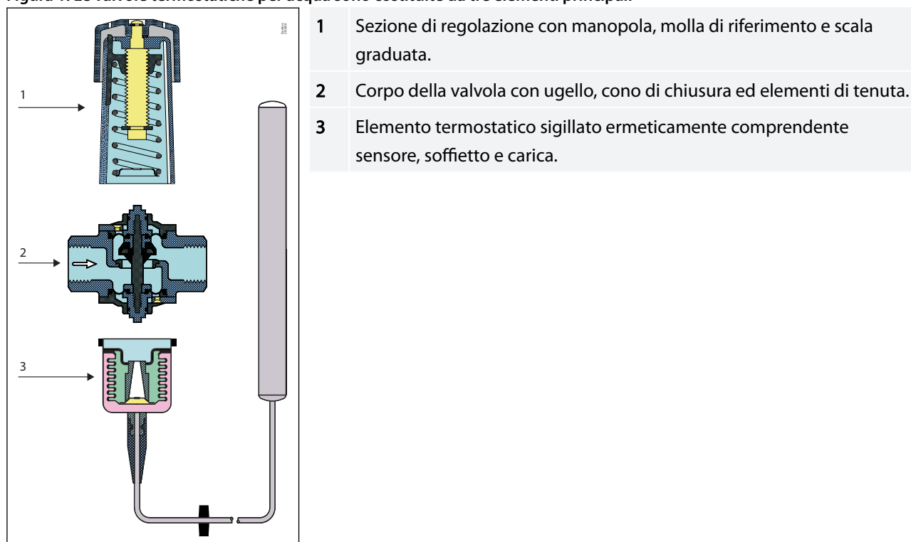
Figura 1: Le valvole termostatiche per acqua sono costituite da tre elementi principali
