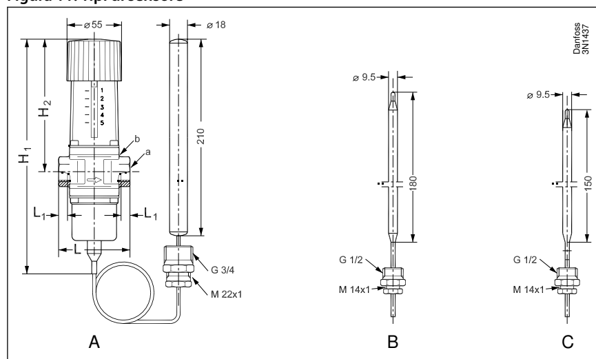
Figura 11: Tipi di sensore
