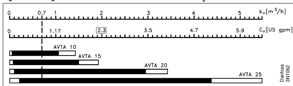
Figura 9: Nomogramma che mostra l'intervallo della valvola k_v
