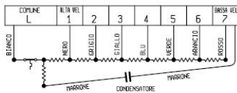
SCHEMA DI COLLEGAMENTO X M02432 E M02434
