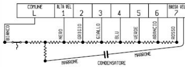
SCHEMA DI COLLEGAMENTO X M02433
