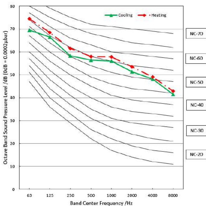
MOX630U-48HFN8-RRD0W(GA)
