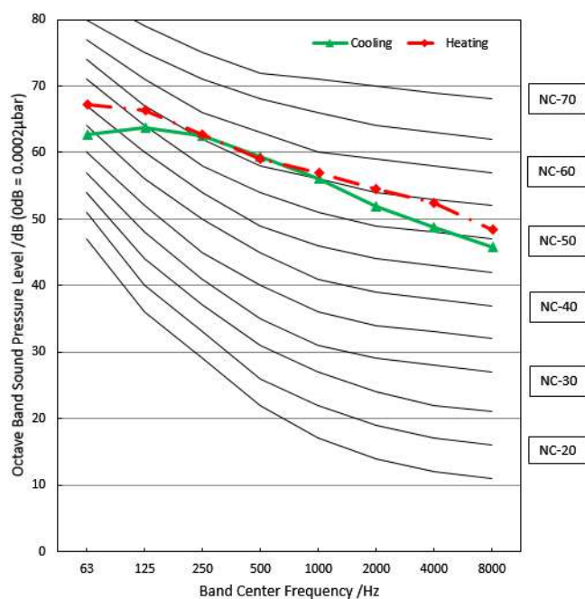
MOD30U-42HFN8-QRD0W(GA)
