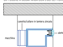
SEZIONE VERTICALE CON VISTA LATERALE DEL DIFFUSORE A SCOMPARSA CON 3 DEFFLETTORI
