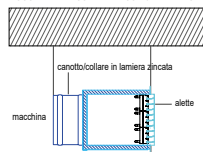
SEZIONE VERTICALE CON VISTA LATERALE DEL BOCCHETTA A SCOMPARSA CON 6 DEFFLETTORI
