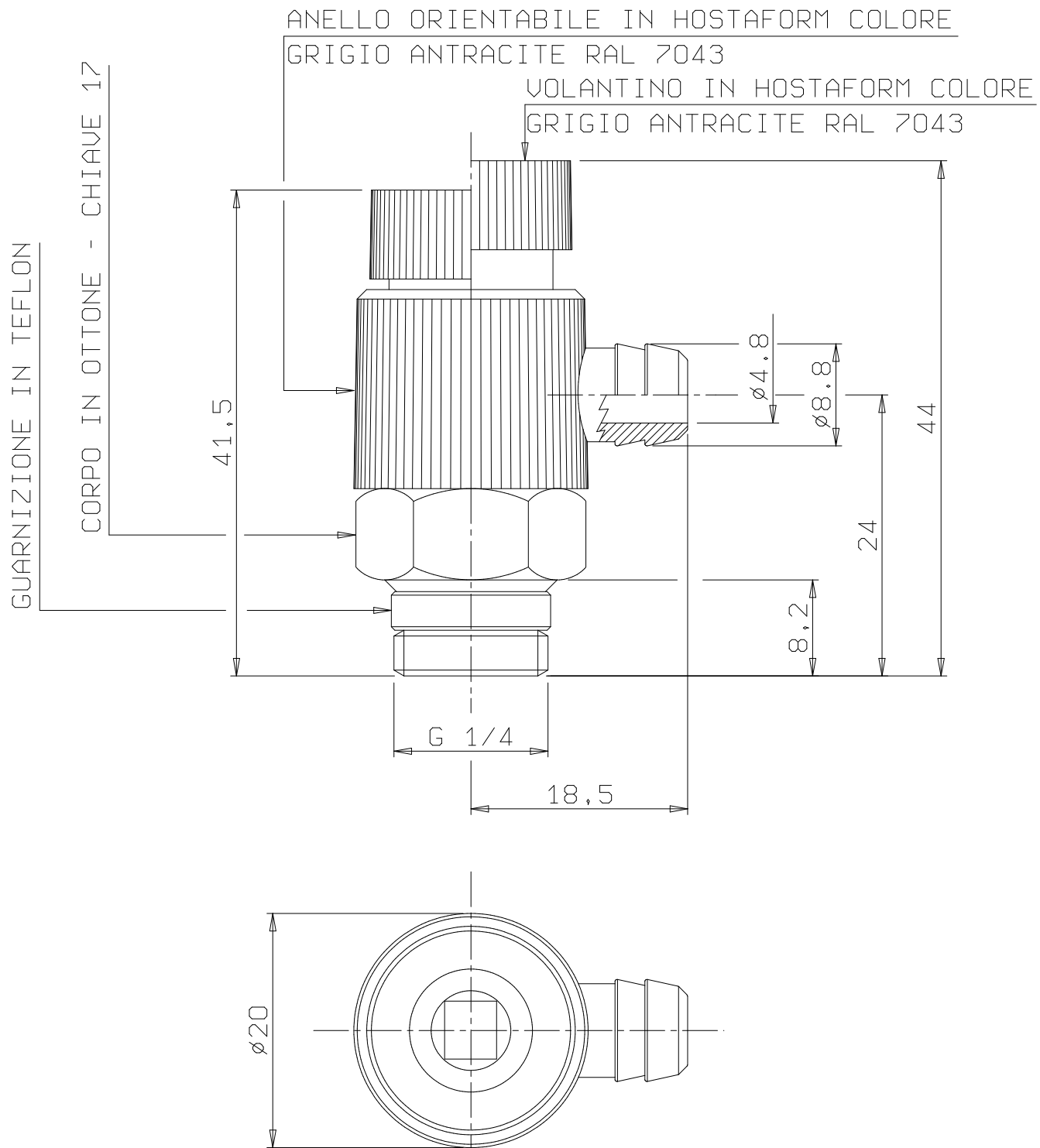
VALVOLA SFIATO ARIA G 1/4 CON ANELLO ORIENTABILE "CALEFFI" ART. 337121
