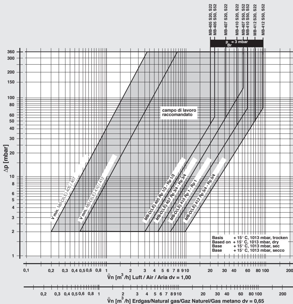
Curva caratteristica della differenza di pressione del flusso volumetrico allo stato regolato con filtro fine
