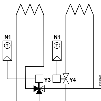
Valvola di zona
