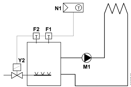
Bruciatore atmosferico
