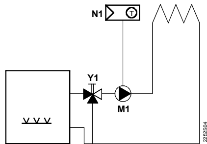
Pompa di circolazione con pre-controllo e valvola di miscela manuale
