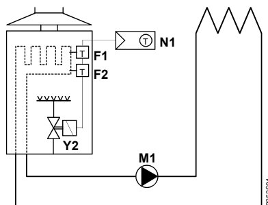
Caldaia murale
