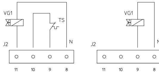
(5a) con termostato di sicurezza (5b) senza termostato di sicurezza
