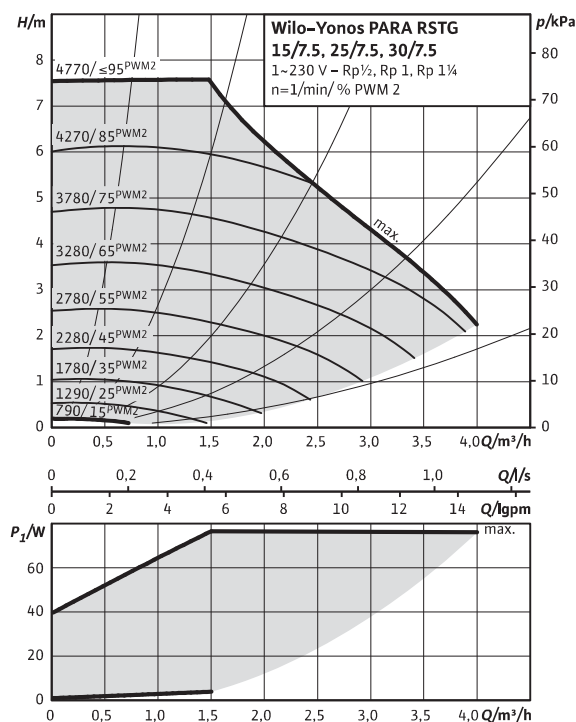
Wilo- RSTG 15/7.5, 25/7.5, 30/7.5
