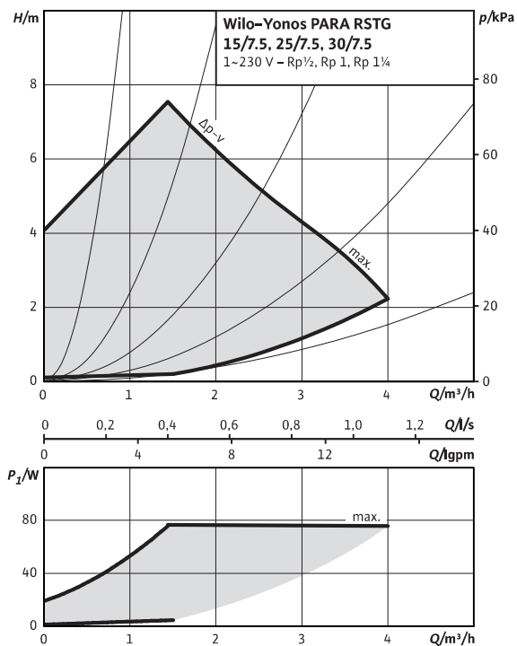
Wilo- RSTG 15/7.5, 25/7.5, 30/7.5
